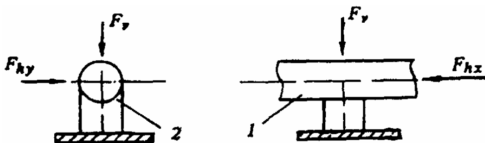
Схема нагрузок на опору
